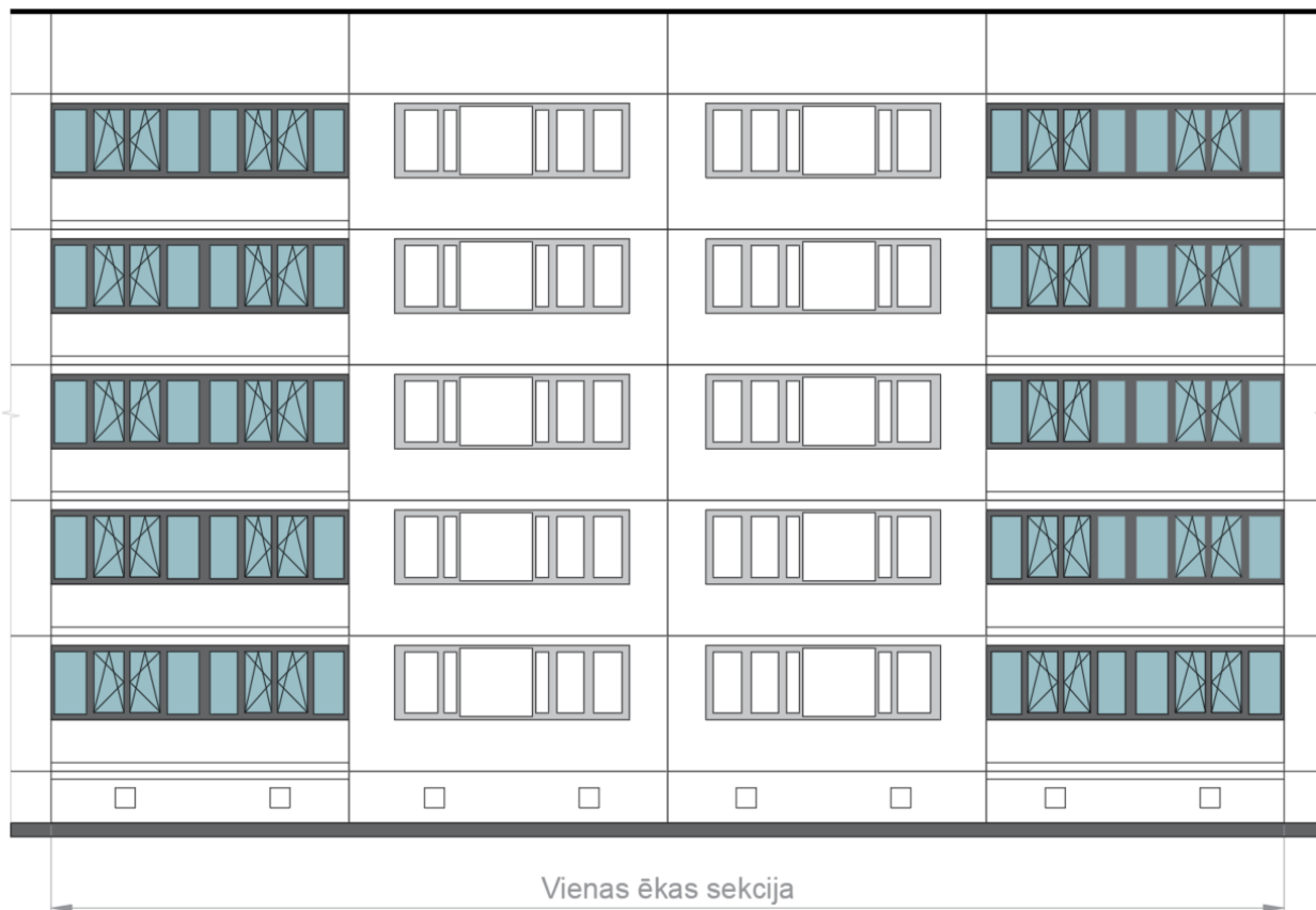
Fasādes shēma
