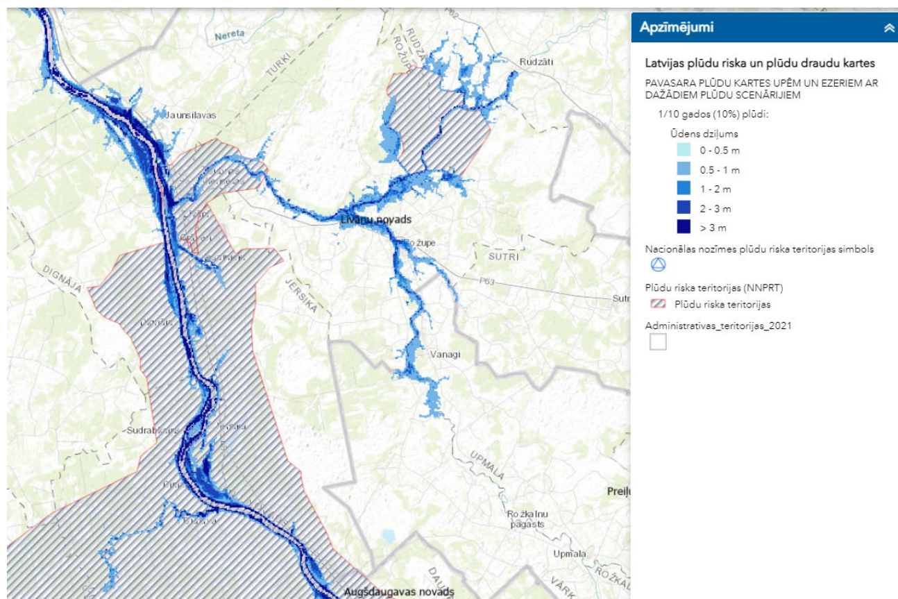
11.8. attēls. Applūstošās teritorijas Datu avots: LVGMC, 2024
